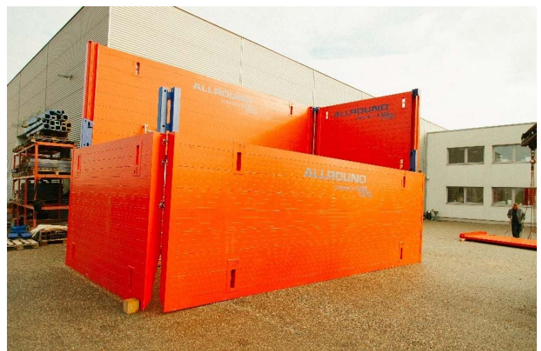
ALU šachtové paženie (dĺžka 7200 x šírka 3600 x výška 4800) pri hmotnosti len od 6 ton.
